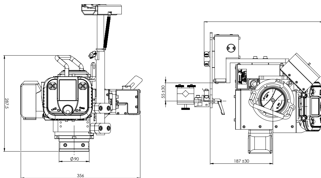
ROTOMAG
